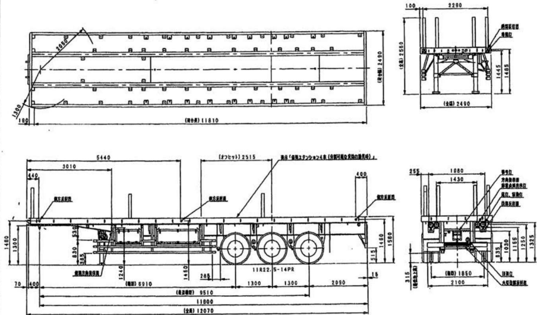
セミトレーラ外観四面図
